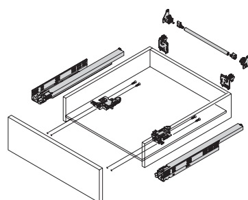
► Tiroir à trois faces
