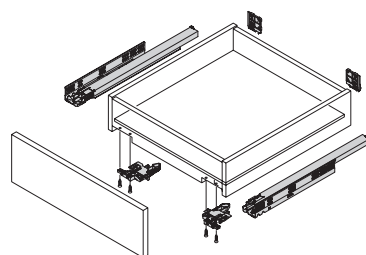
► Tiroir à quatre faces
