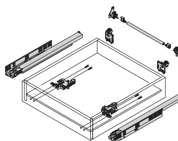
► Tiroir à l'anglaise
