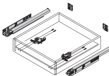
► Tiroir à l'anglaise
