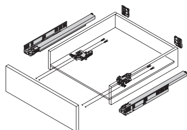
► Tiroir à trois faces
