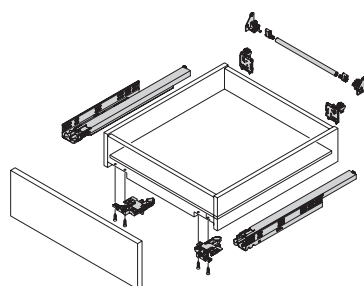
► Tiroir à quatre faces
