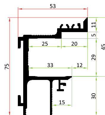
Profils de châssis TUS50
