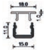
60.110.59 Abbildung mit Endkappe und Befestigungsclip
