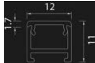
60.188.03 Abbildung mit Endkappe
