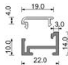
60.188.18-24 Abbildung mit Endkappe
