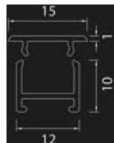
60.110.55 Abbildung mit Endkappe und Befestigungsclip
