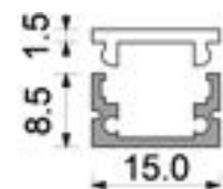
60.188.05 Abbildung mit Endkappe
